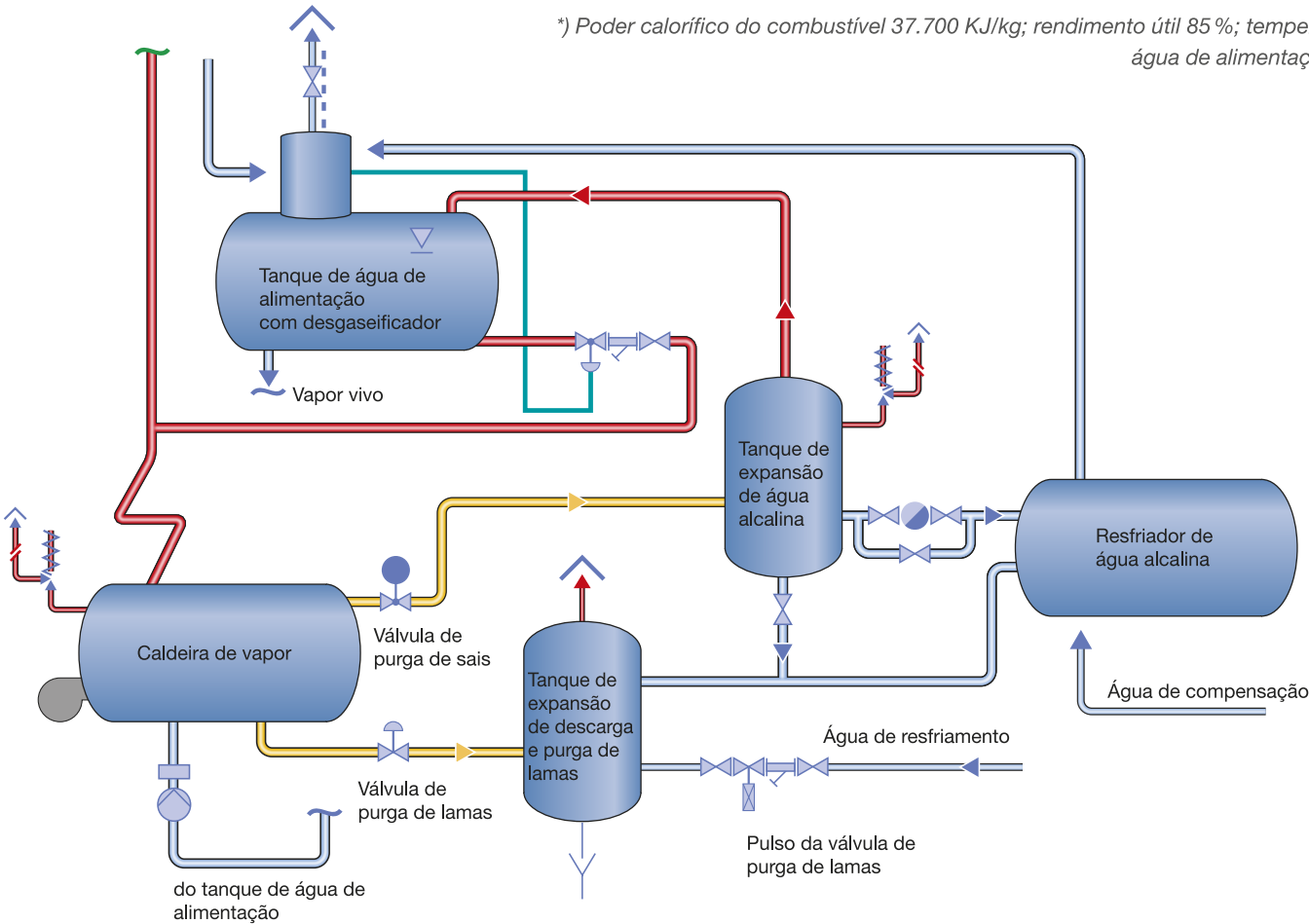
Esquema de um sistema de expansão de água alcalina com tanque de expansão de descarga e de purga de lamas
